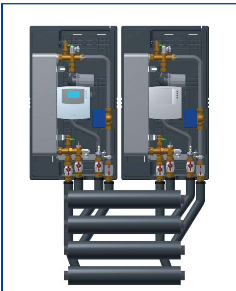
Frischwasserstation MULTIFRESH Master- und Slavestation
